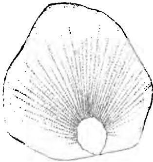
Fig. 11. Fremdstrahlung um ein Bläschen aus Niederschlagsmembran. Zelle aus einem mit 2\frac{1}{2} -proc., eben saurer Albumoselösung imprägnirten Hollundermarkprisma, das 20 Std. in ALTMANN's Bichromat-Osmiumgemisch gelegen hatte. Dieses Fixirungsmittel gibt sehr schöne Niederschlagsmembranen, von denen eine sich bläschenförmig in das Zellumen vorgewölbt hat. Die Oberfläche dieser Niederschlagshaut hat als Wecker für die Strahlungen gedient, über deren Entstehung man den beifolgenden Text vergleichen wolle. Das sehr engmaschige Gerüstwerk, das die Strahlungsfigur umschliesst, besteht aus der übrigen, feinglobulitisch ausgefällten Albumose. (Vergr. 330.)
